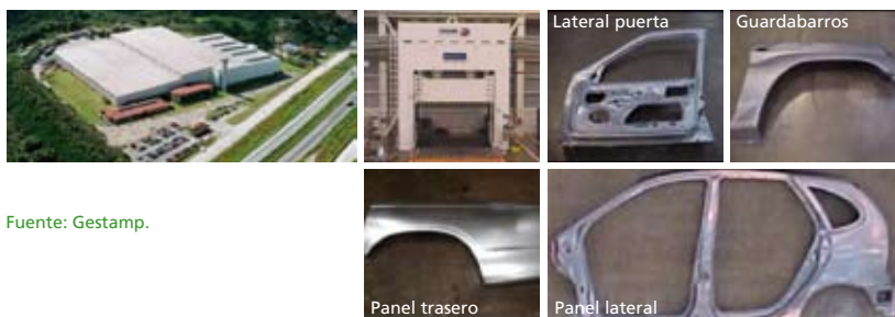
Gráfico 8: Planta de Paraná y productos fabricados
